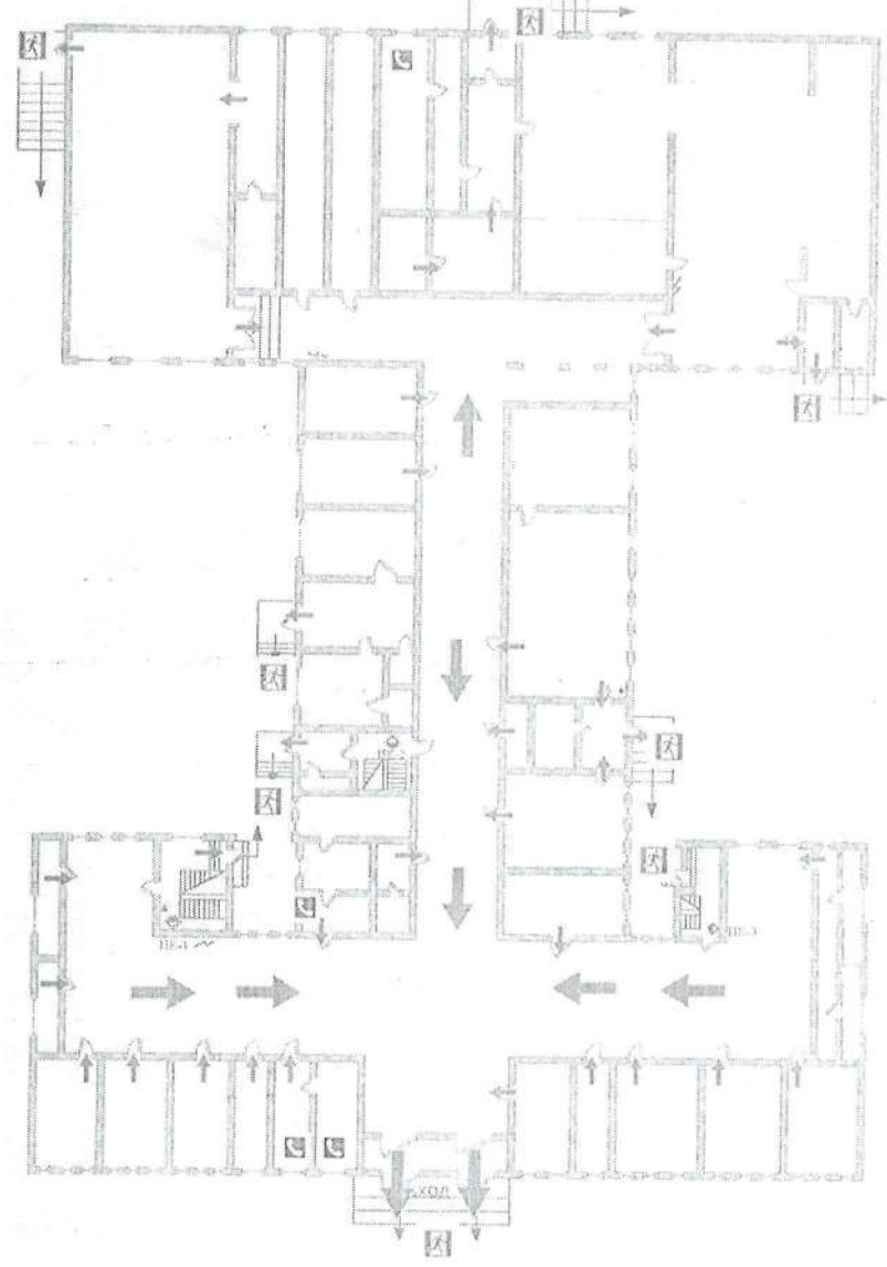
План эвакуации при угрозе совершения или совершении террористического акта 1 этаж
